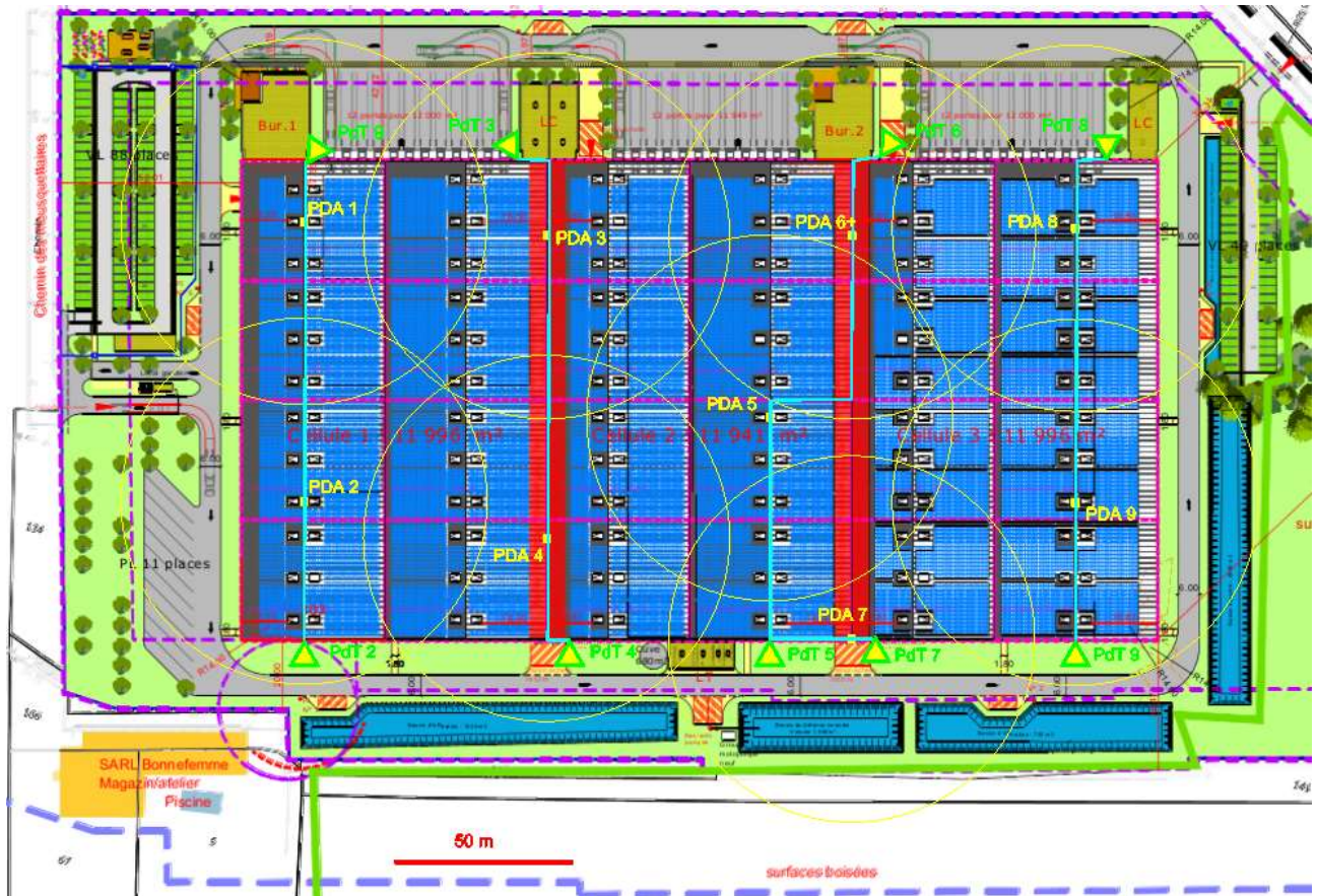
Plan 5: Implantation des paratonnerres, conducteurs de descente et prises de terre
