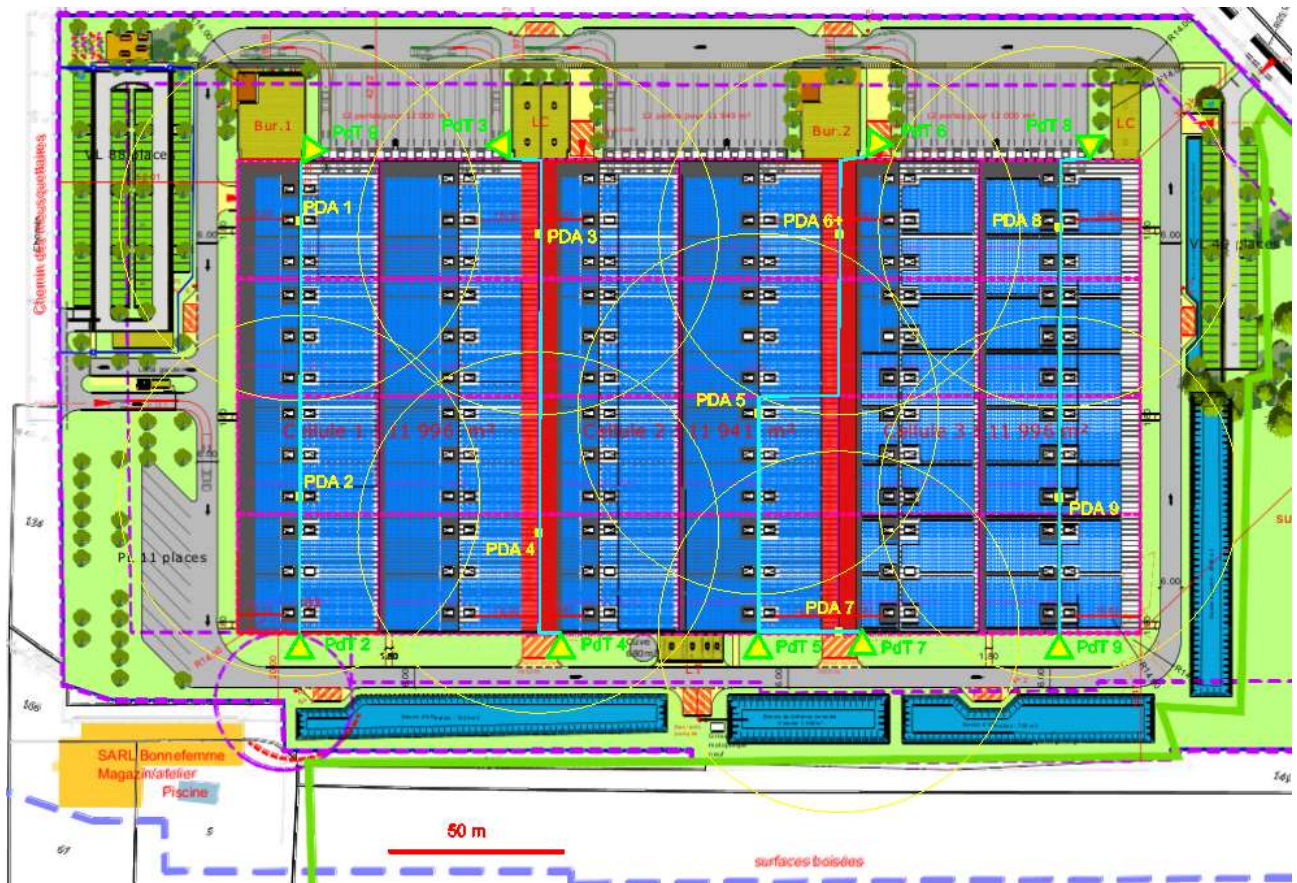
Plan 6: Implantation des paratonnerres, conducteurs de descente et prises de terre
