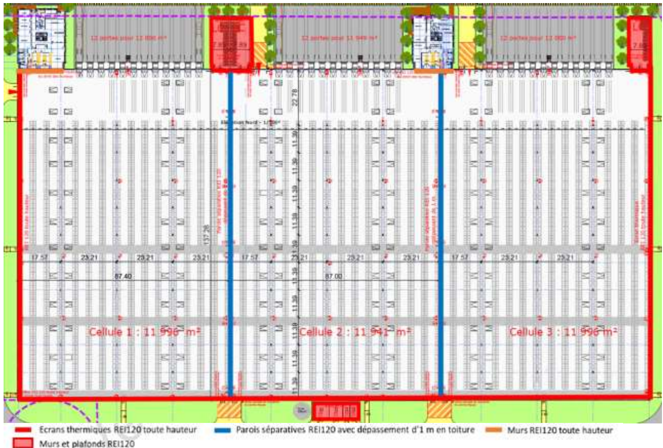
Plan 4 : Murs coupe-feu de l'entrepôt
