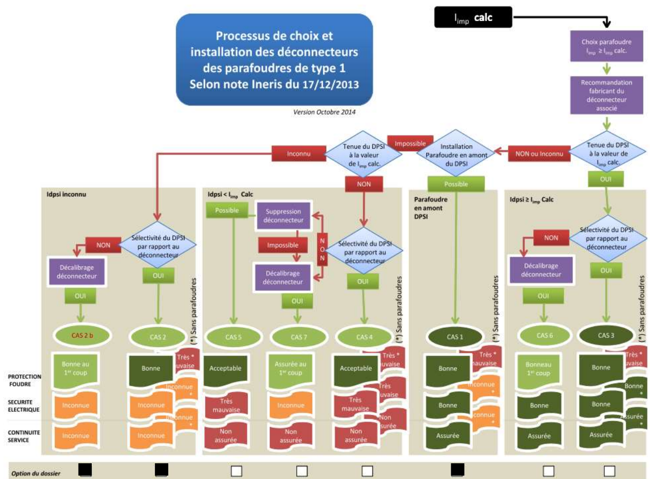
Figure 11 : Dispositifs de déconnection des parafoudres de type 1
